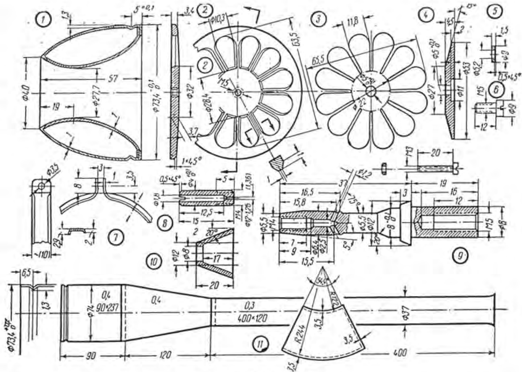
Рис. 63. ПуВРД Аэроджет-2:
